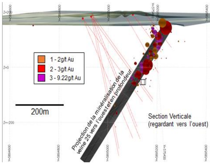
Figure 2. Section verticale regardant vers l'ouest, montrant les traces de forage proposées en rouge par rapport aux extensions possibles de la Zone 25 (polygone gris).
