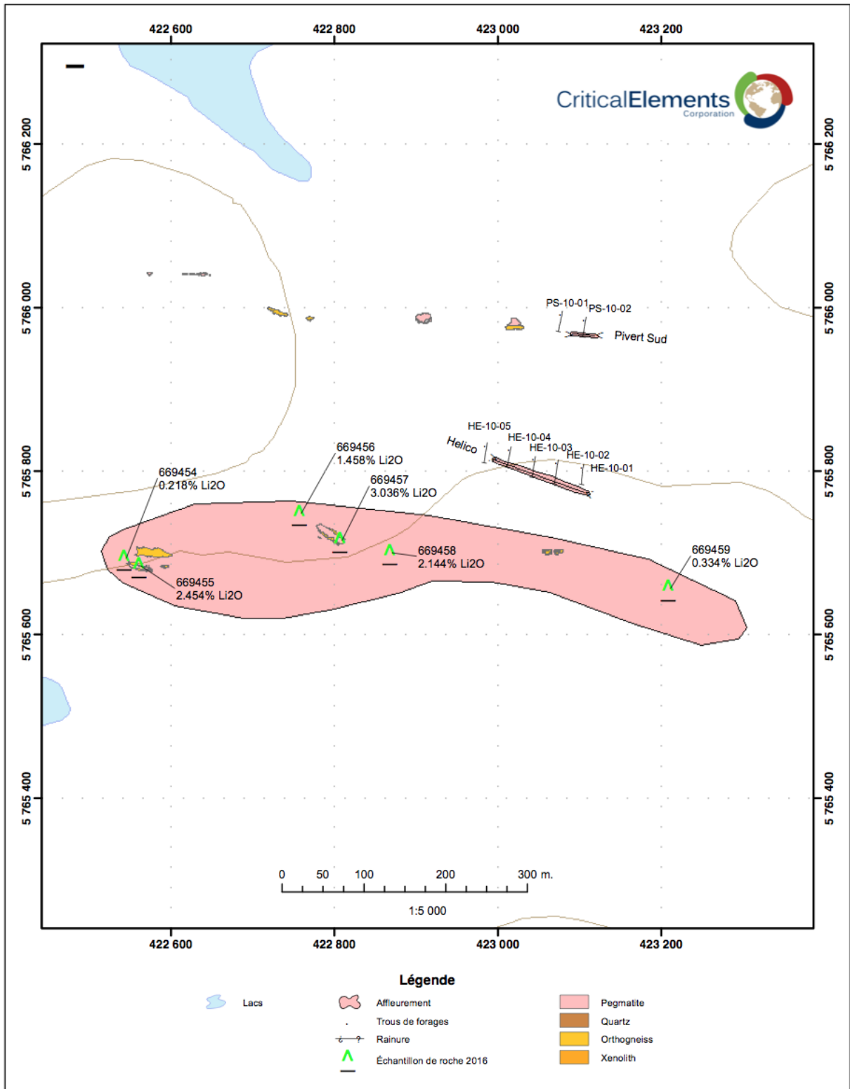
Figure 2. Carte de localisation des échantillons recueillis sur l'indice Helico-Sud
