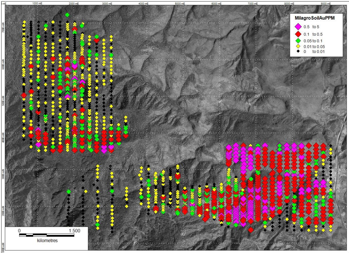
Anomalie en or de géochimie de sols à Milagro
