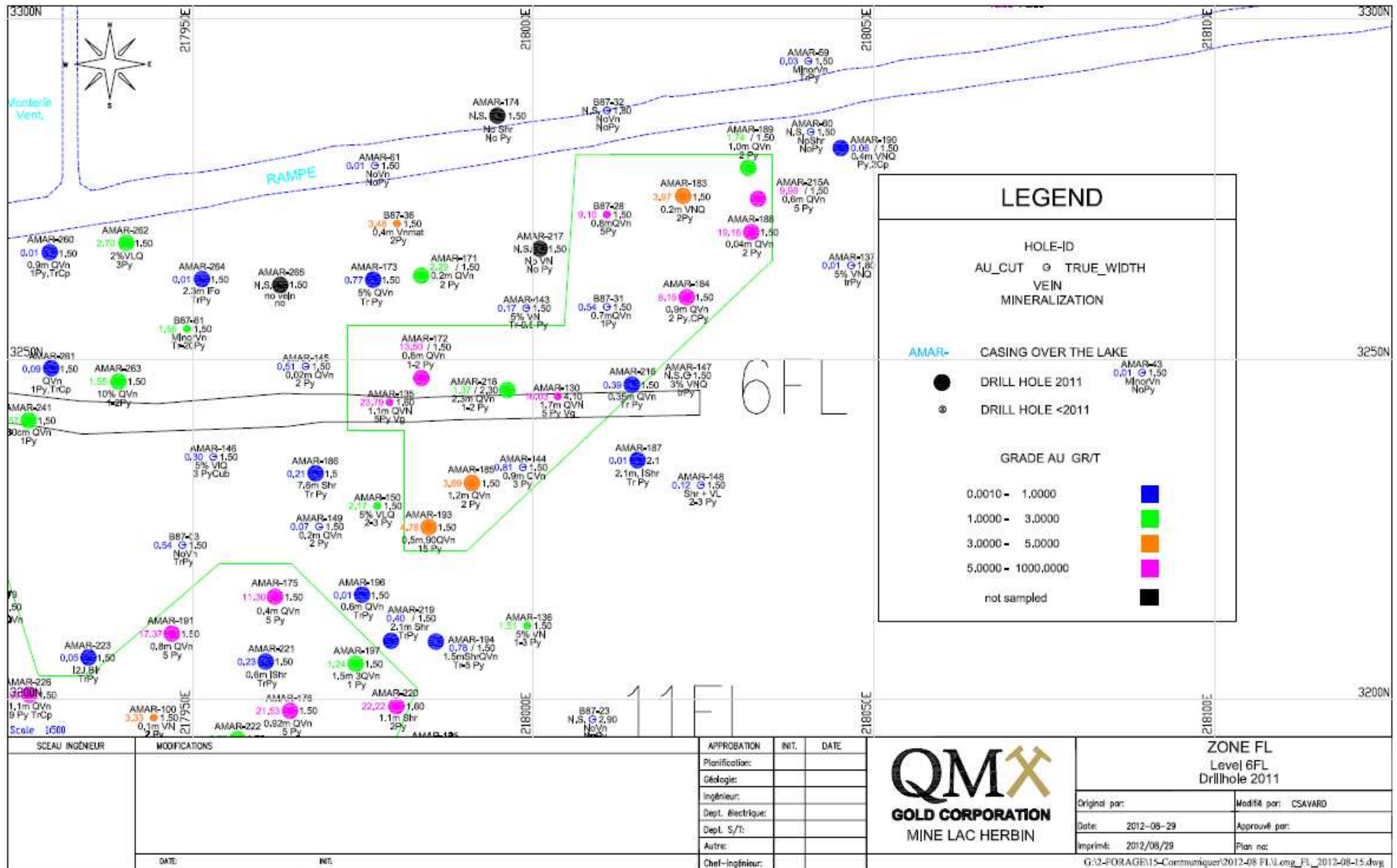
Figure 2 : Zone FL — Section longitudinale 6 FL
