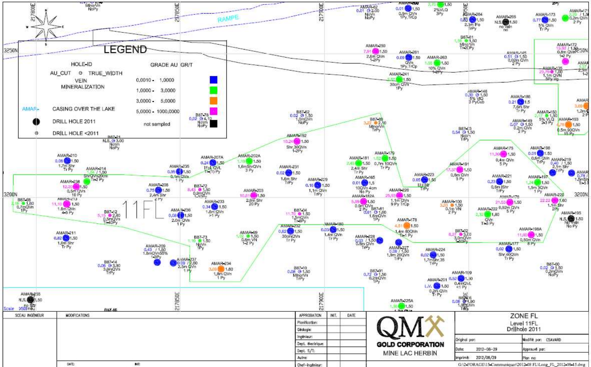
Figure 3 : Zone FL — Section longitudinale 11 FL
