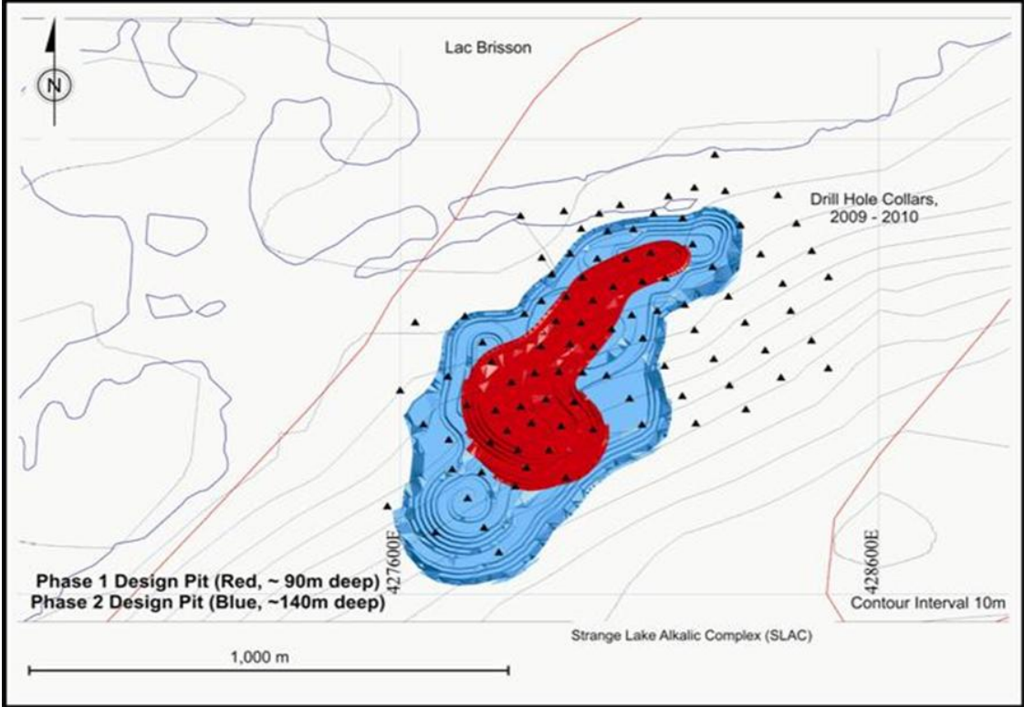
Figure 4: Phase 1 et phase 2 du design de la mine
