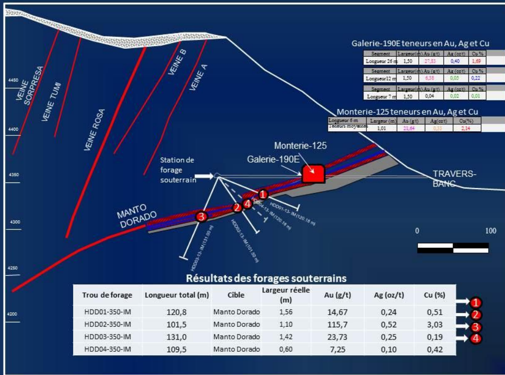
Figure 1. Forages souterrains HDD01-2013 à HDD-04-2013, Manto Dorado, Tumipampa.
