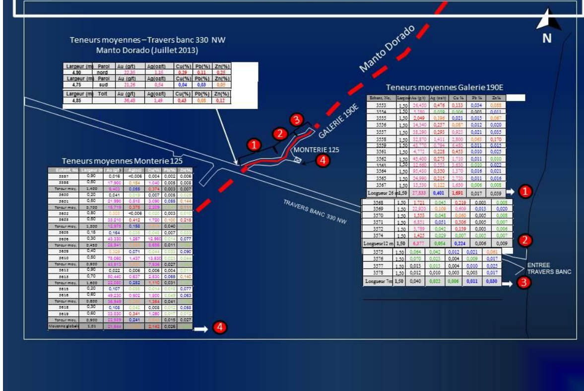
Figure 2 Plan de l'excavation souterraine, du travers-banc, de la galerie et de la monterie, Manto Dorado, Tumipampa.
