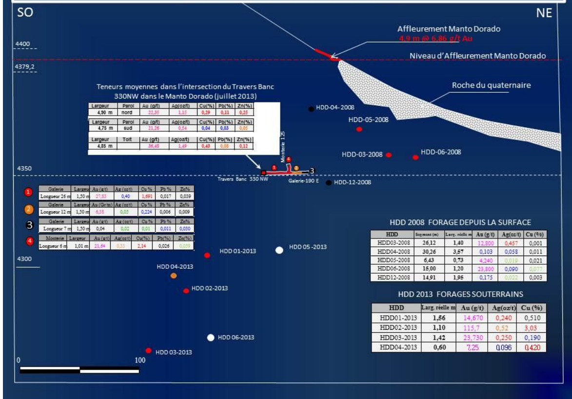
Figure 3. Section longitudinale des forages, du travers-banc, de la galerie et de la monterie et résultats de l'échantillonnage, Manto Dorado, Tumipampa.
