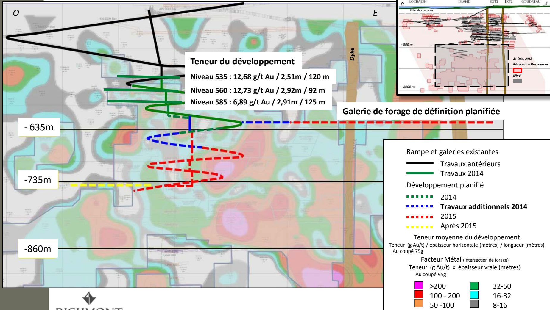
Section Longitudinale Composite
