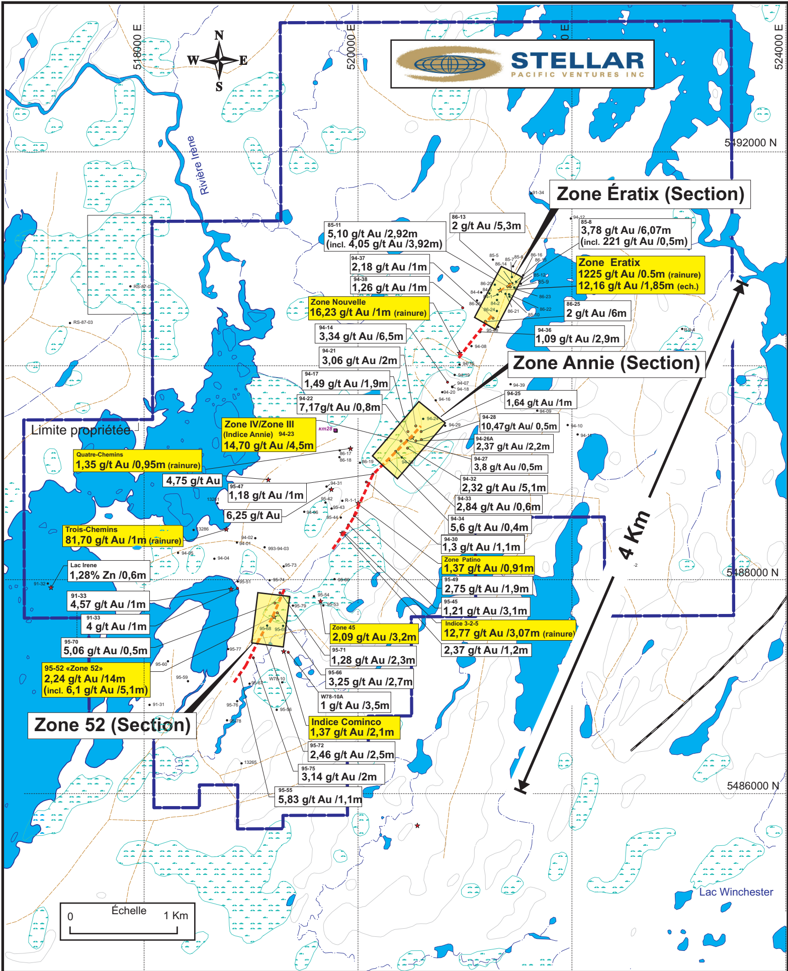
PRINCIPAUX INDICES AURIFÈRES - PROJET LAC AU MONSTRE
