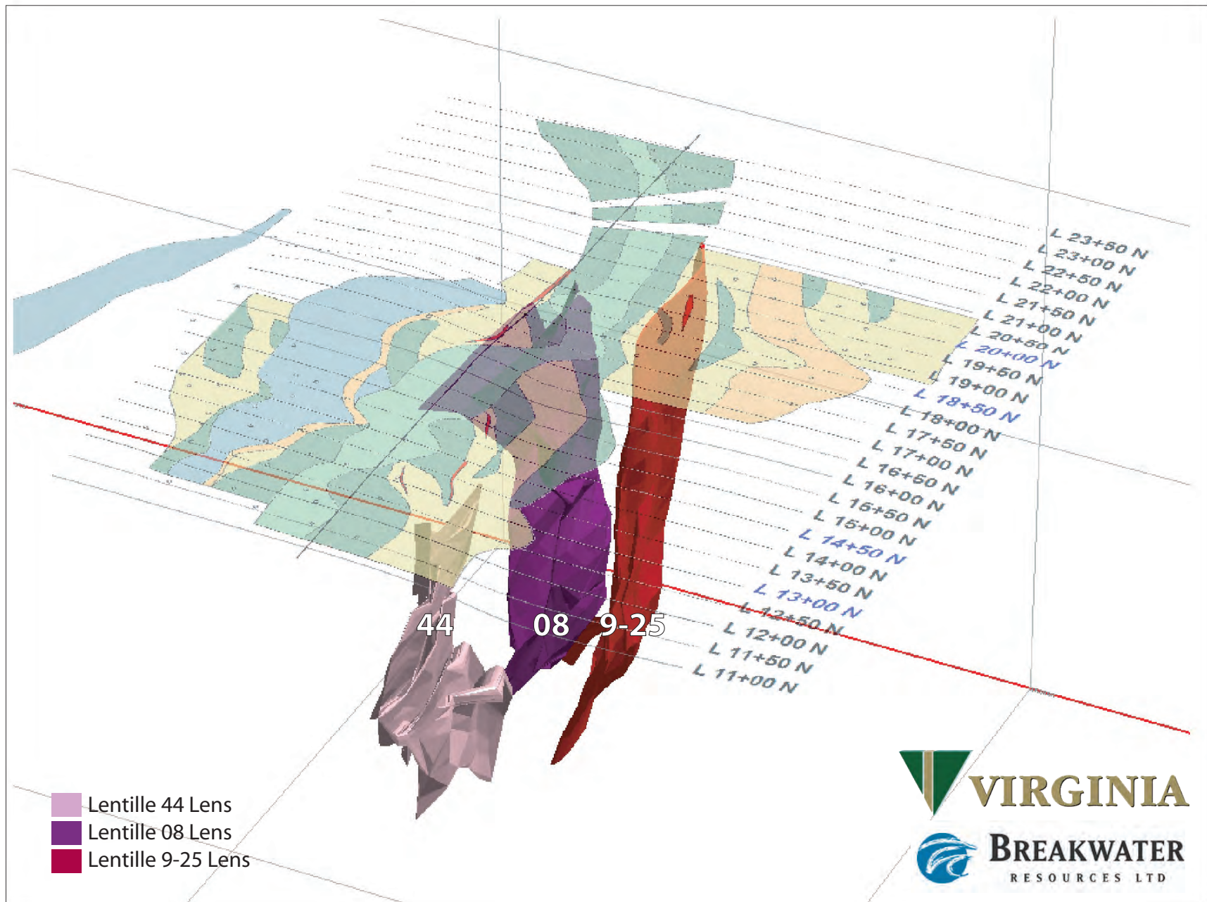
Vue en 3D vers le Nord-Ouest avec géologie de surface 3D view looking northwest with surface geology
