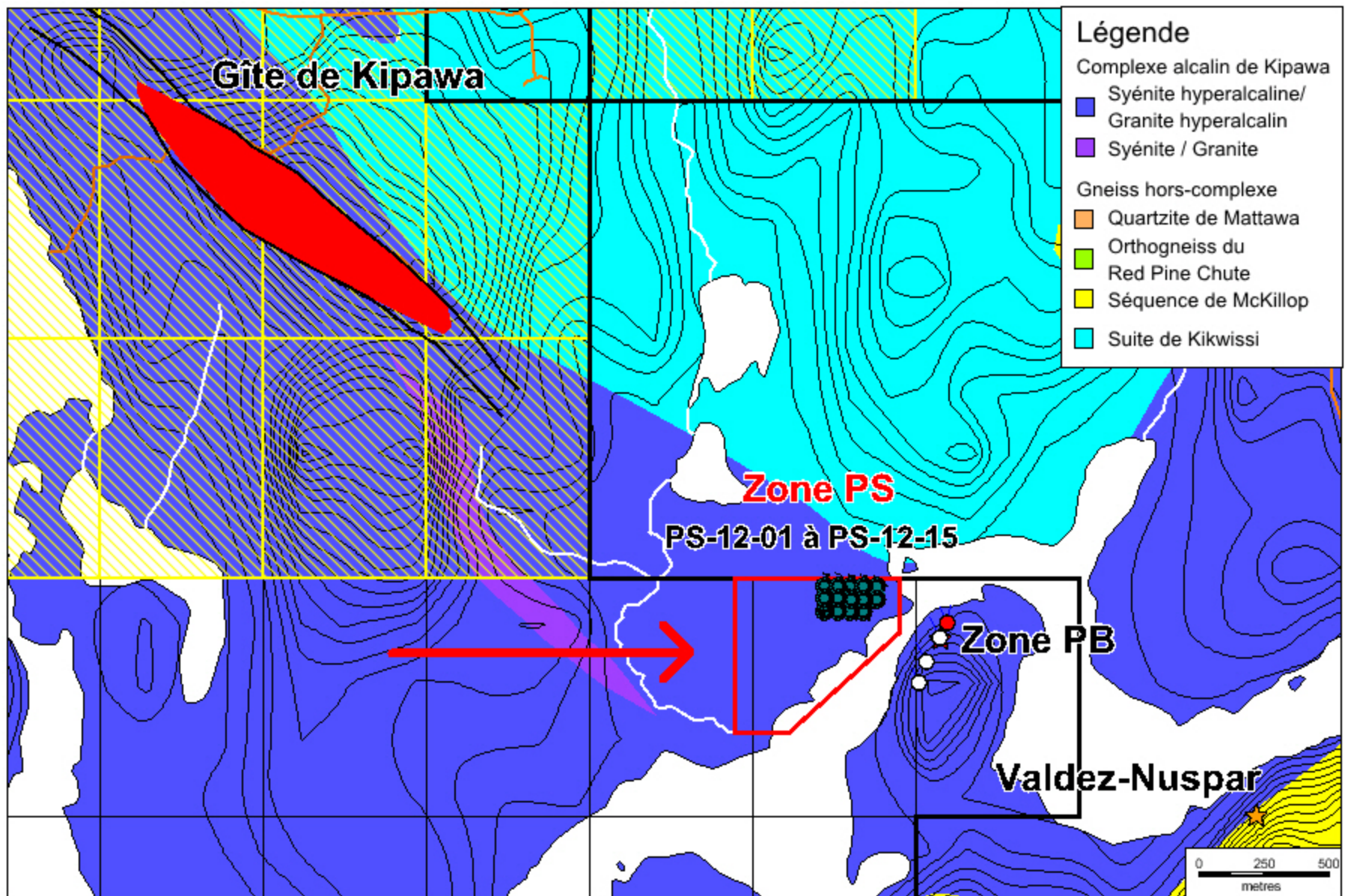
Figure 1 : Localisation des sondages sur la zone PS de Matamec Explorations inc. Les sondages forés par Unocal en rouge (sondage minéralisée) et blanc (sondages non minéralisés). Les titres miniers de la co-entreprise en jaune.
