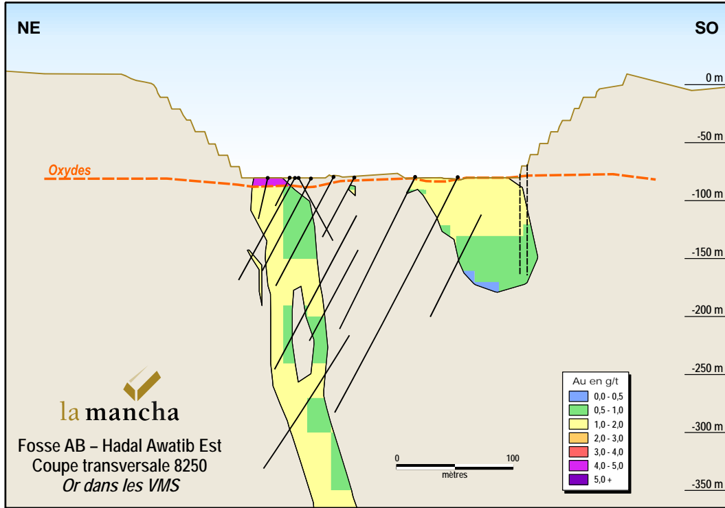
Figure 2a Coupe transversale 8250 – Or dans les VMS
