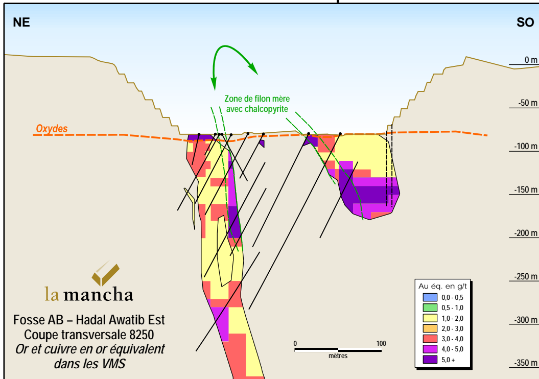
Figure 2b Coupe transversale 8250 – Or et cuivre en or équivalent dans les VMS
