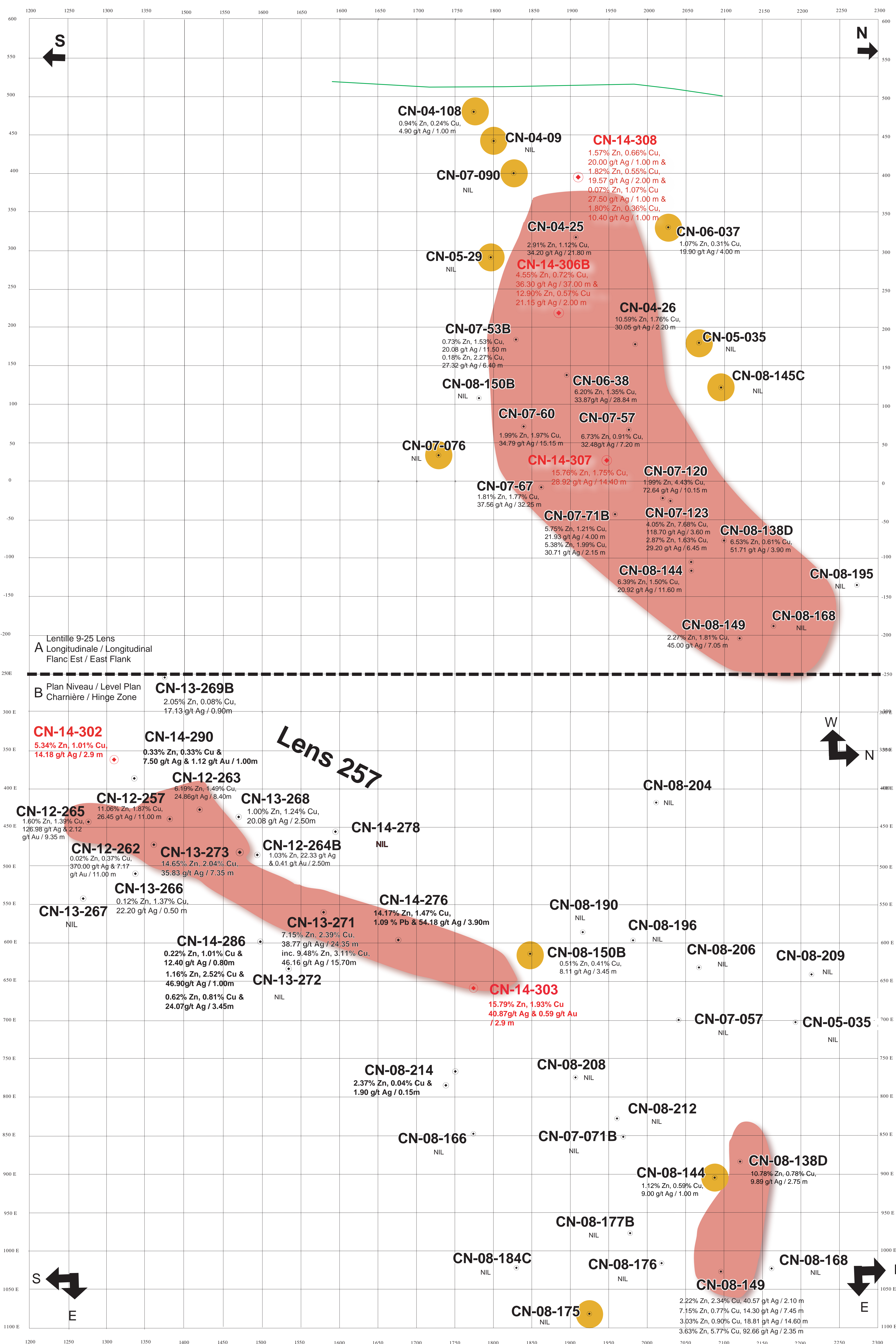
Longitudinal Section Lens 9-25 & Plan View Lens 257 / Section Longitudinale Lentille 9-25 & Vue en Plan Lentille 257
