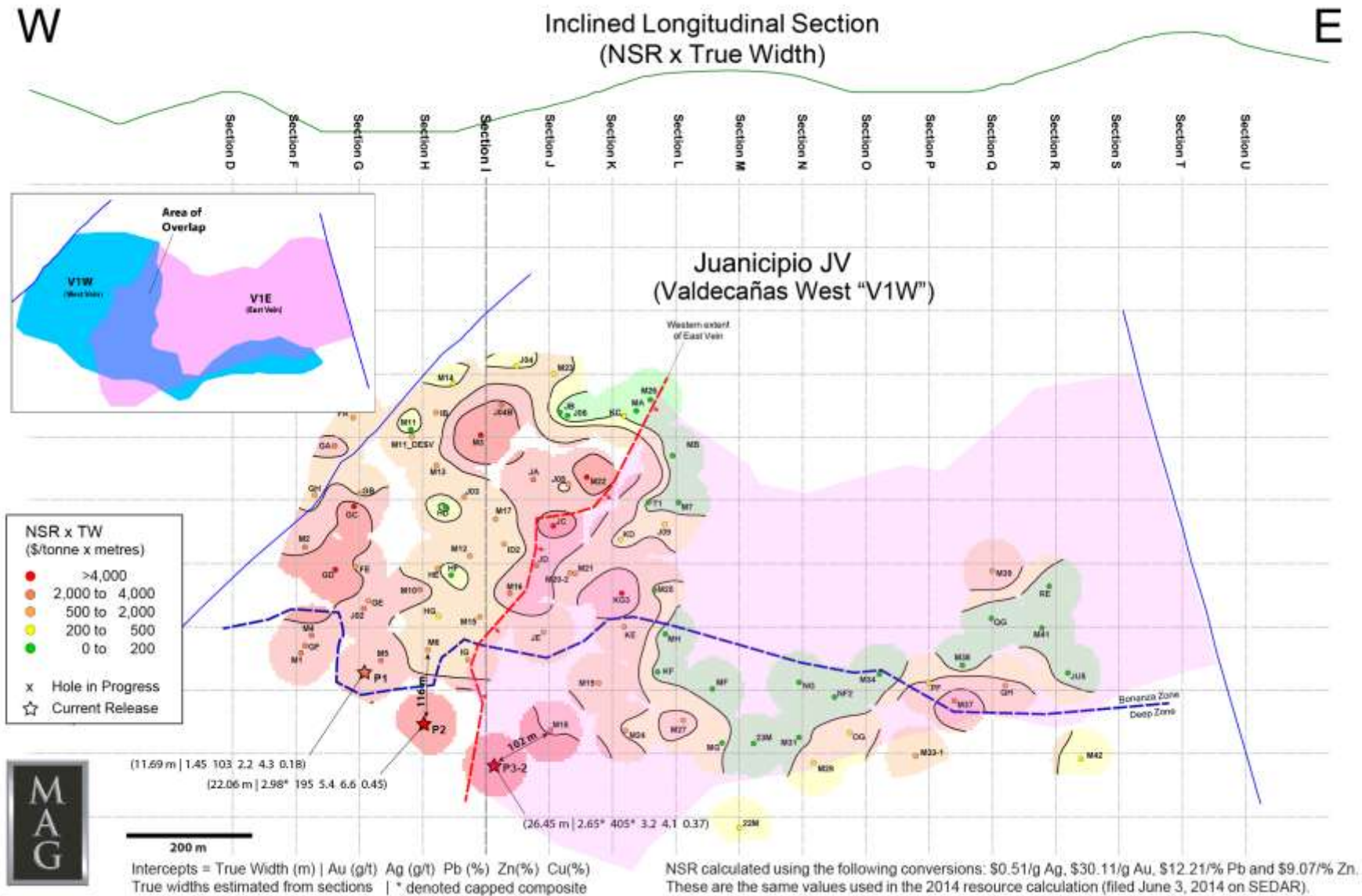
Figure 2: Minera Juancipio, Valdecañas West- Longitudinal Section
