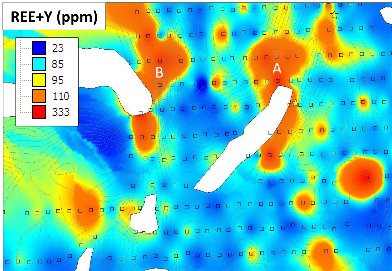
FIGURE 2. ANOMALIES DE SOL, HORIZON B, RÉGION INDICE SURPRISE (Carrés=stations aux 100m, Étoiles=indices, Lignes=courbes de niveaux aux 5m)
