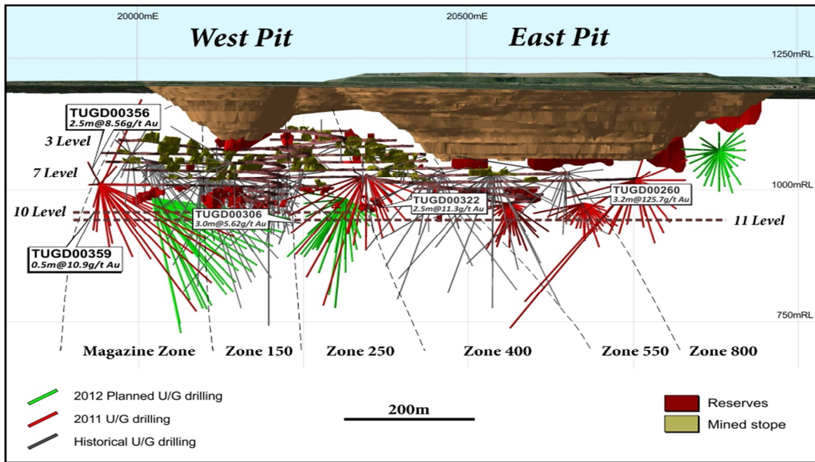
Figure – Section longitudinale montrant les meilleures intersections du forage en dessous du 7e niveau
