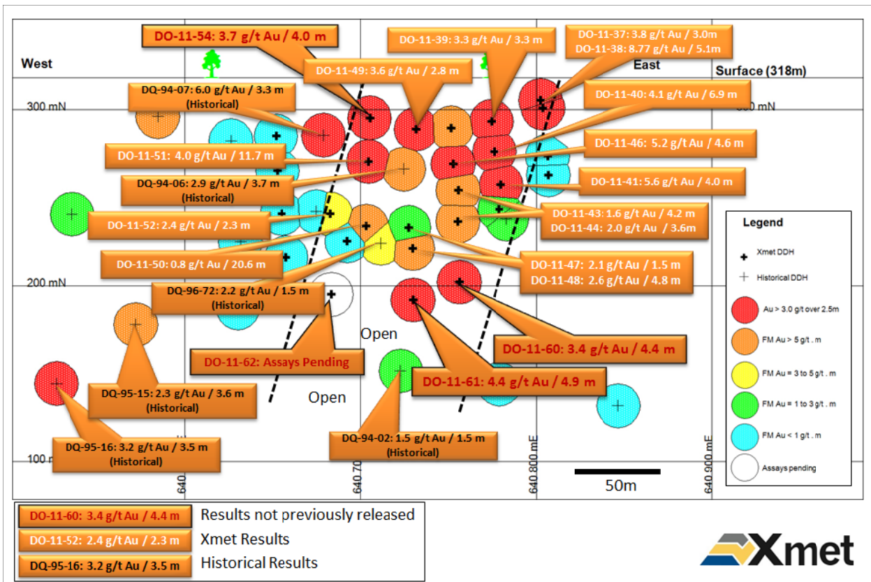
Figure 1 : Section longitudinale montrant la partie est de la zone Shaft située à faible profondeur sur la propriété Duquesne-Ottoman. Toutes les longueurs sont des intervalles dans l'axe de forage et les épaisseurs réelles minéralisées représentent environ 80 % des longueurs dans l'axe de forage.
