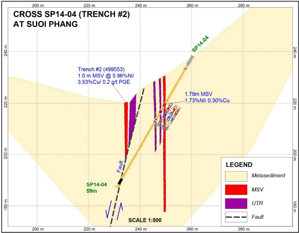
Figure 5. Suoi Phang Geological Interpretation.
