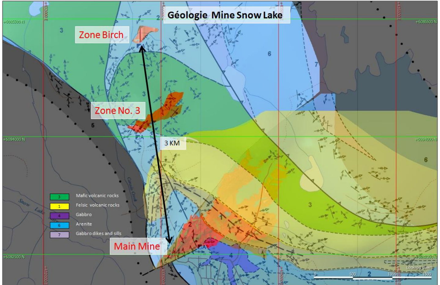
Figure 1: La géologie de la mine Snow Lake et la position relative de Birch, Zone No. 3, et la Zone Main Mine
