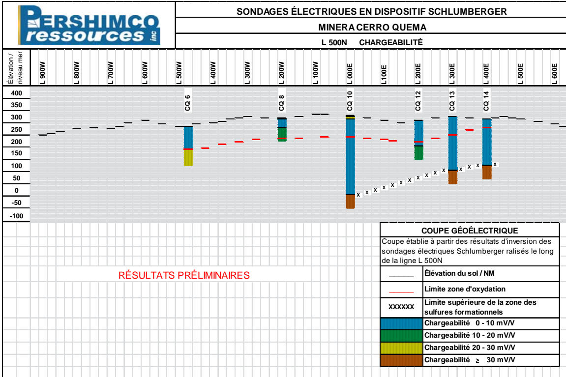
Figure 1 : résultats préliminaires de l'inversion des Sondages Électriques, TL 5+00N.
