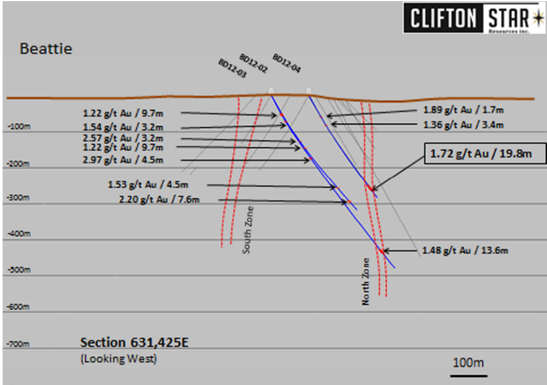
SECTION 631,425E
