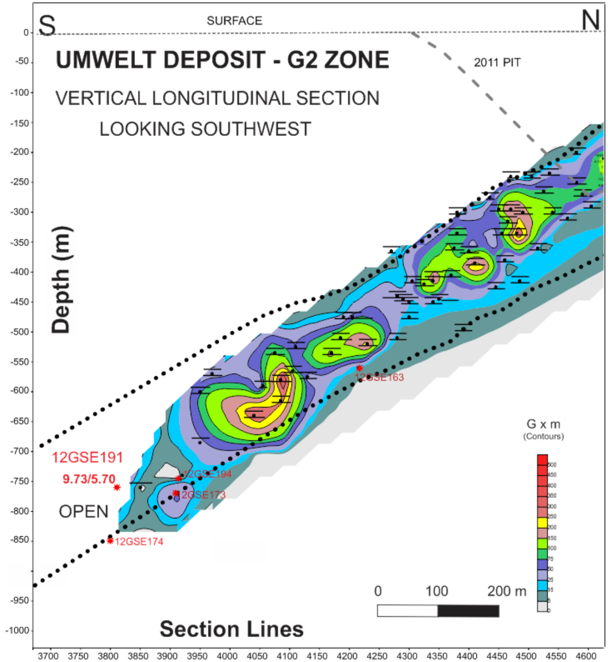
Figure 2: Umwelt G2 Longitudinal section
